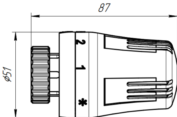
Рисунок 1 – Габаритные размеры
